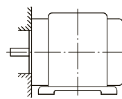
IM B34
