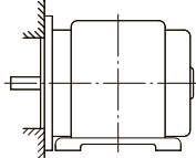
IM B35
